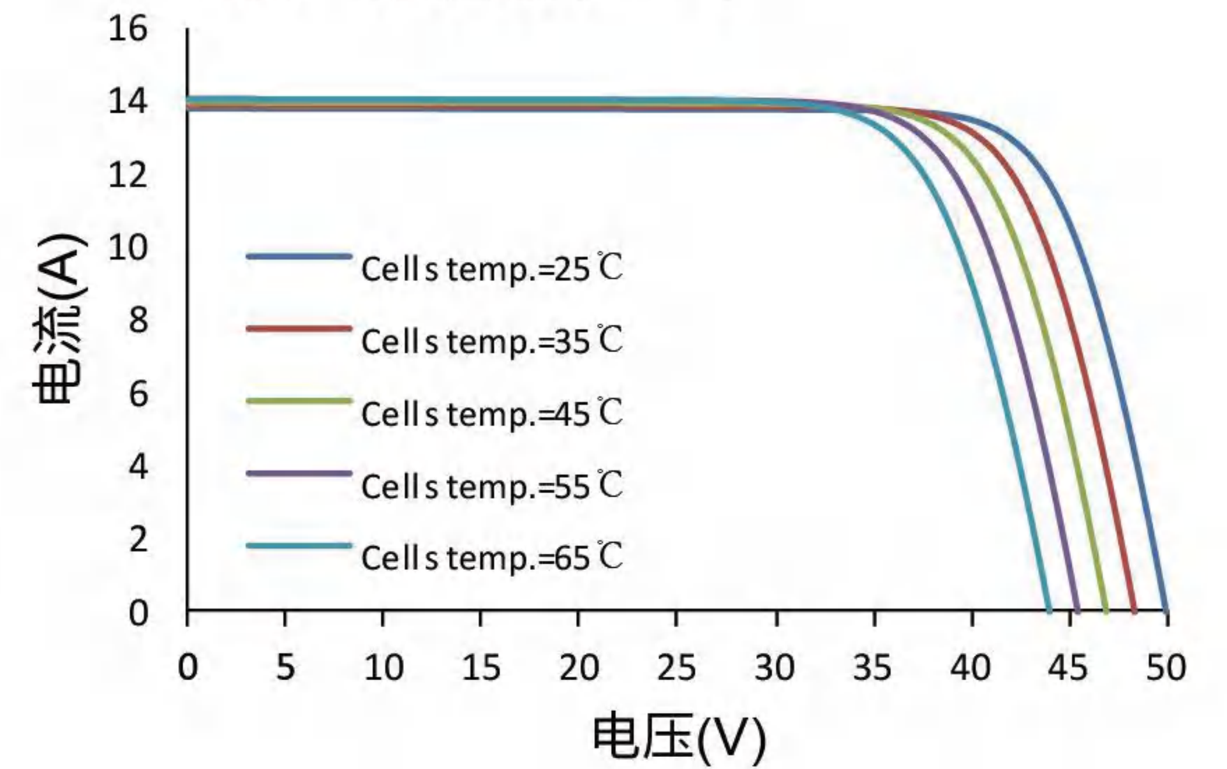
电流-电压曲线 (545W)
