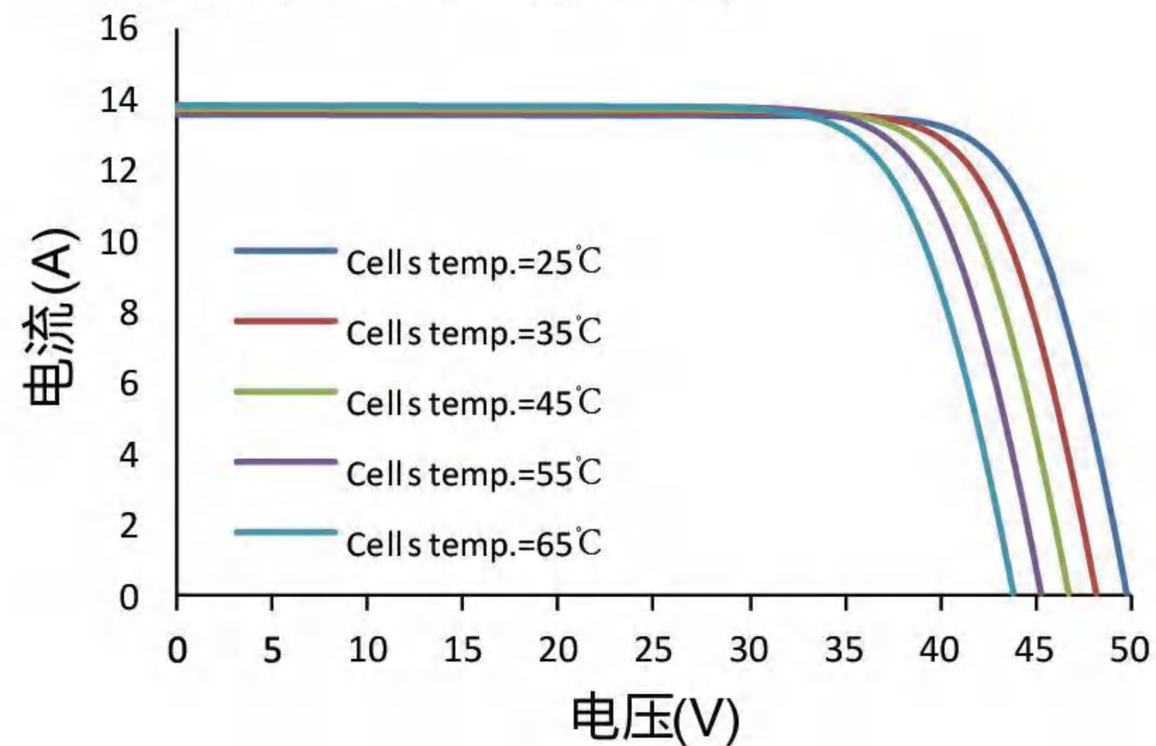
电流-电压曲线 (540W)
