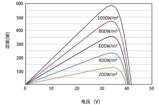
组件的P-V曲线 (590W)
