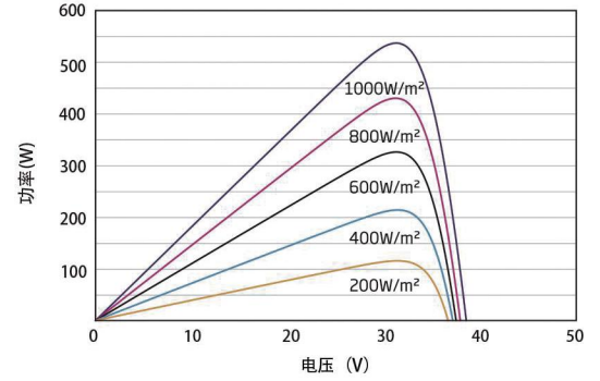
组件的P-V曲线
